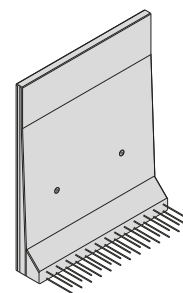
Pied avec armature saillante
